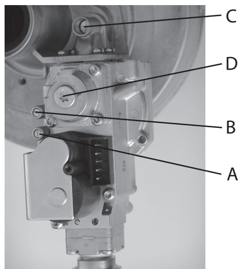
Obr. 4.3.6: Prvky pre meranie a nastavenie plynovej armatúry Honeywell VK 4125
